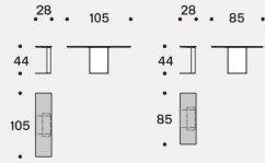
MYT 1&2 (esempio SX / Left example)
